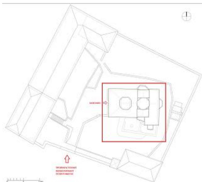
Εικ. 2 Κάτοψη μοναστηριακού συγκροτήματος: το καθολικό τοποθετείται περίπου στο μέσον της αυλής. (Αρχιτεκτονική μελέτη στερέωσης και αποκατάστασης, ΓΕΑΜ Μνημείο ΕΠΕ, 2024)
